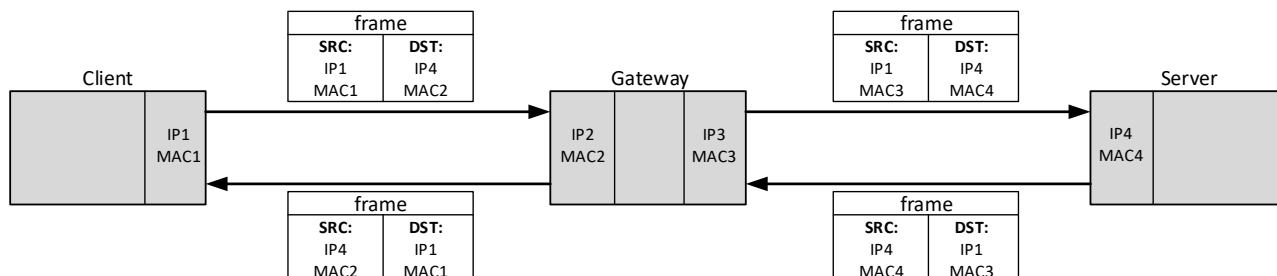
Рисунок 6.5. Пример прохождения кадров при запросе из другой подсети
